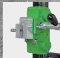
Attacco della macchina: portautensili universale
